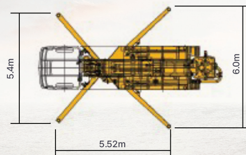
아우트리거 펼침거리
