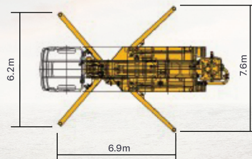
아우트리거 펼침거리
